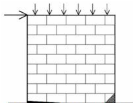
Vlačno popuštanje (lijevo) i tlačno drobljenje pete zida (desno) - „savijanje“
