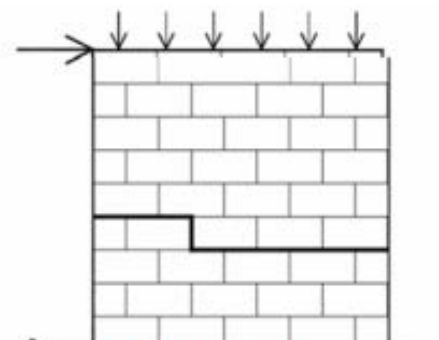
Posmični slom „klizanje“
