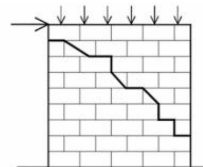
Vlačni slom (ili posmični) „dijagonalni slom“
